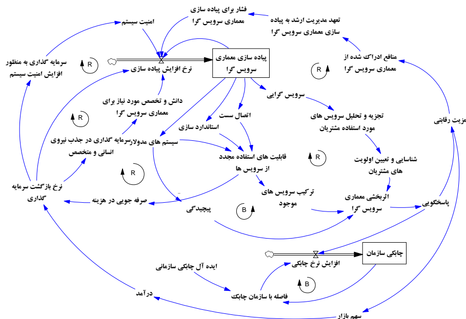
شکل ۴: مدل مفهومی تحقیق در قالب نمودار انباشت و جریان
