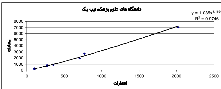
نمودار ۲. رابطه بین تولیدات علمی و استنادات دانشگاه‌های علوم پزشکی تیپ یک
