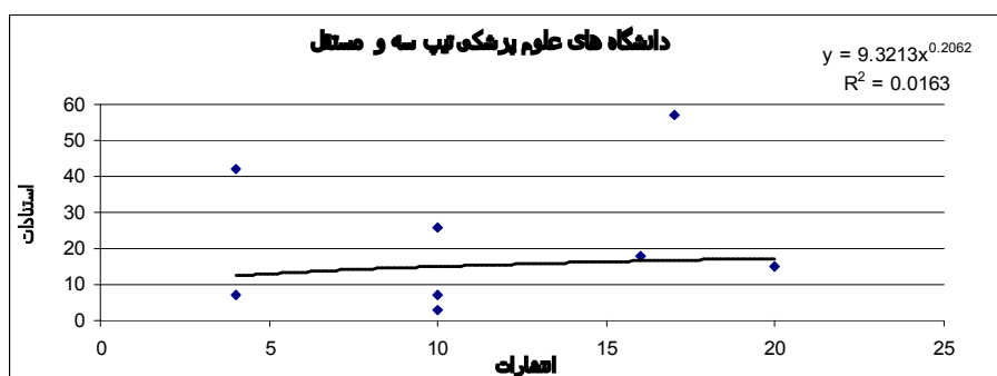
نمودار ۴. رابطه تولیدات علمی و استنادات دانشگاه‌های علوم پزشکی تپ سه و مستقل
