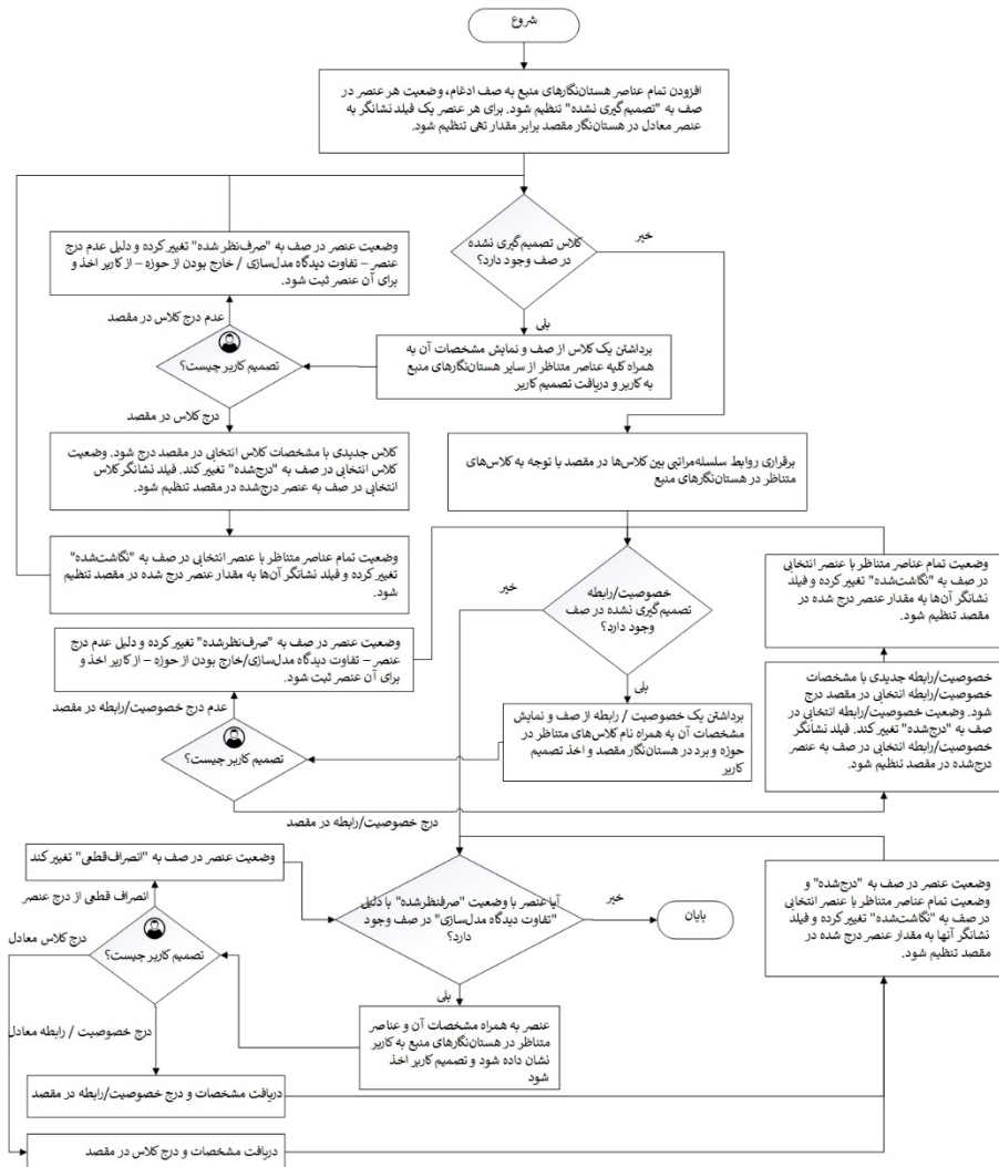
شکل ۵. الگوریتم ادغام هستان‌نگارها
