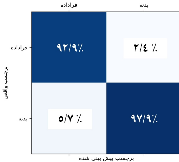
شکل ۸. ماتریس درهم‌ریختگی
