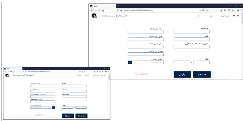
شکل ۸. رابط کاربری موتور جست‌وجوی پیشرفته درگاه جست‌وجوی یکپارچه مخازن سازمانی ایران (آیریس)
