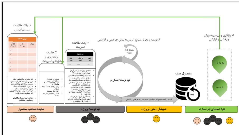
شکل ۴. چگونگی فرایند طراحی و توسعه درگاه جست‌وجوی یکپارچه مخازن سازمانی ایران با استفاده از چارچوب «چابک اسکر ام»
