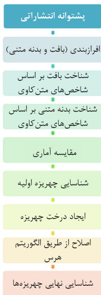
شکل ۲. الگوریتم پیشنهادی
