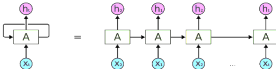
تصویر ۱. عملکرد شبکه‌های عصبی بازگشتی (Olah 2015)
