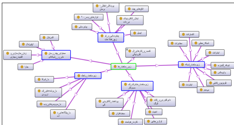
شکل ۷. آنوگراف کلاس‌ها و زیرکلاس‌های مفهومی رده زیرساخت‌های کسب‌وکارهای الکترونیک
